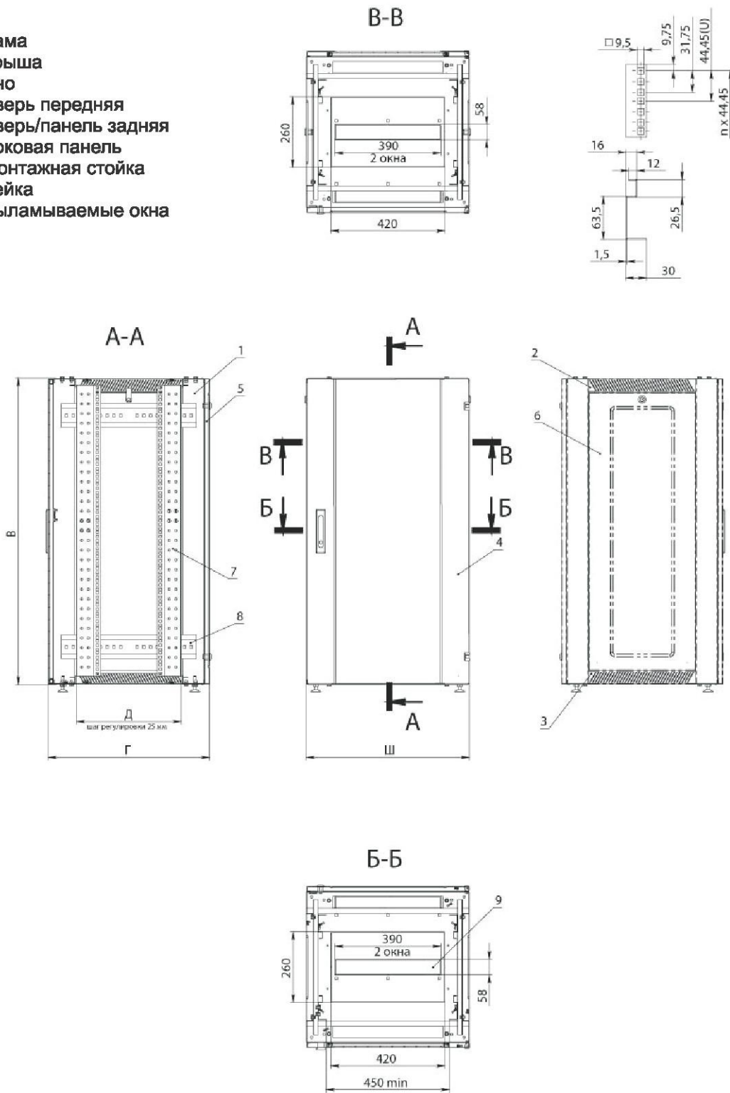
Схема шкафов серии С
